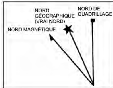
Figure 12-2-1 Trois nords
